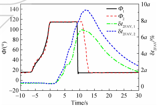
图 7 起飞状态保持时间对发动机进口温度畸变强度的影响 Fig. 7 Effect of working duration on engine inlet face temperature distortion intensity
