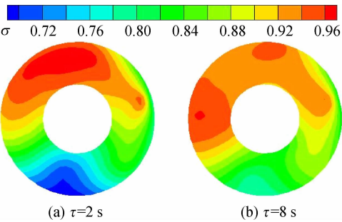
图 5 不同时刻发动机进口总压恢复系数 \sigma 分布云图对比 ( \tau=2 s, \tau=8 s)
