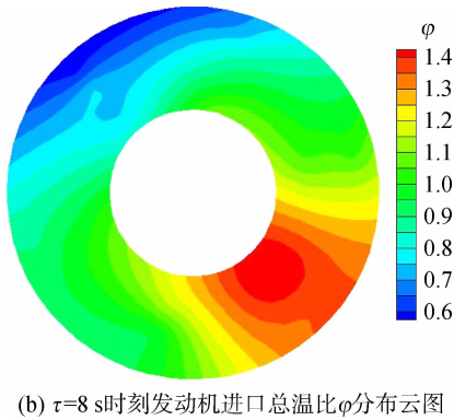
图 3 发动机进口压力和温度分布云图 Fig. 3 Pressure and temperature contours on engine inlet face
