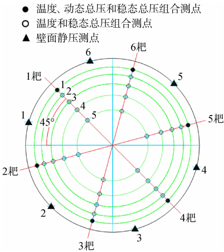
图 1 发动机进口测点布置示意图(逆航向视图)
