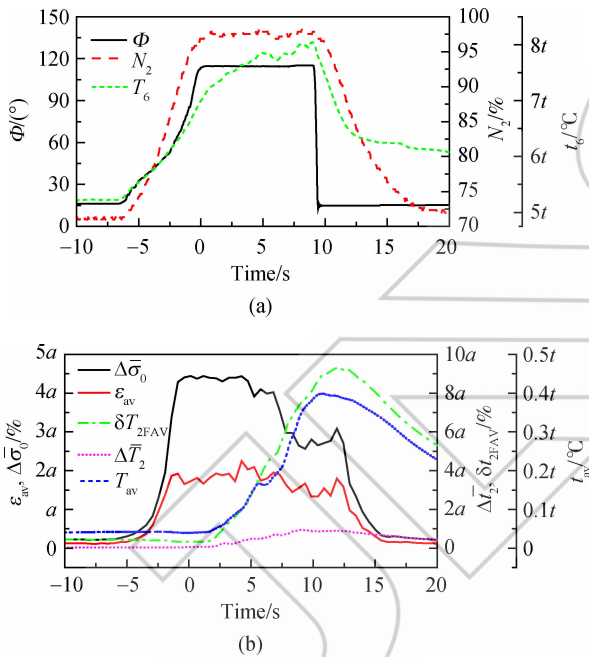
图 2 发动机工作参数和进口流场畸变指数时间历程曲线 Fig. 2 Time history of engine working parameters and inlet flowfield distortion indicators
