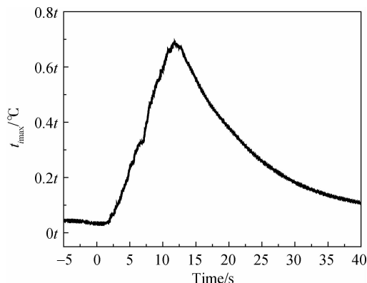
图8 最大温升测点修正后温度历程曲线
