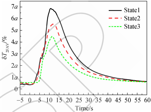
图 6 发动机不同工作状态时进口温度畸变强度 Fig. 6 Temperature distortion intensity in different engine thrust levers
